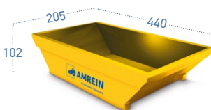
Normal-Mulde 7.0 m 3
