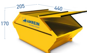
Mulde gedeckt 10.0 m 3
