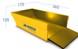
Mulde mit Rückladen 4.0 m 3 (Innenbreite 1.4 m)
