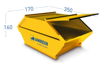
Mulde gedeckt 6.0 m 3
