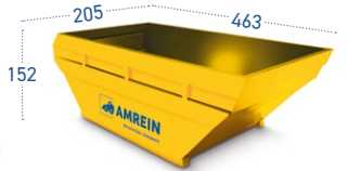
Normal-Mulde 9.0 m 3 (oder Schlamm-Mulde gedeckt)
